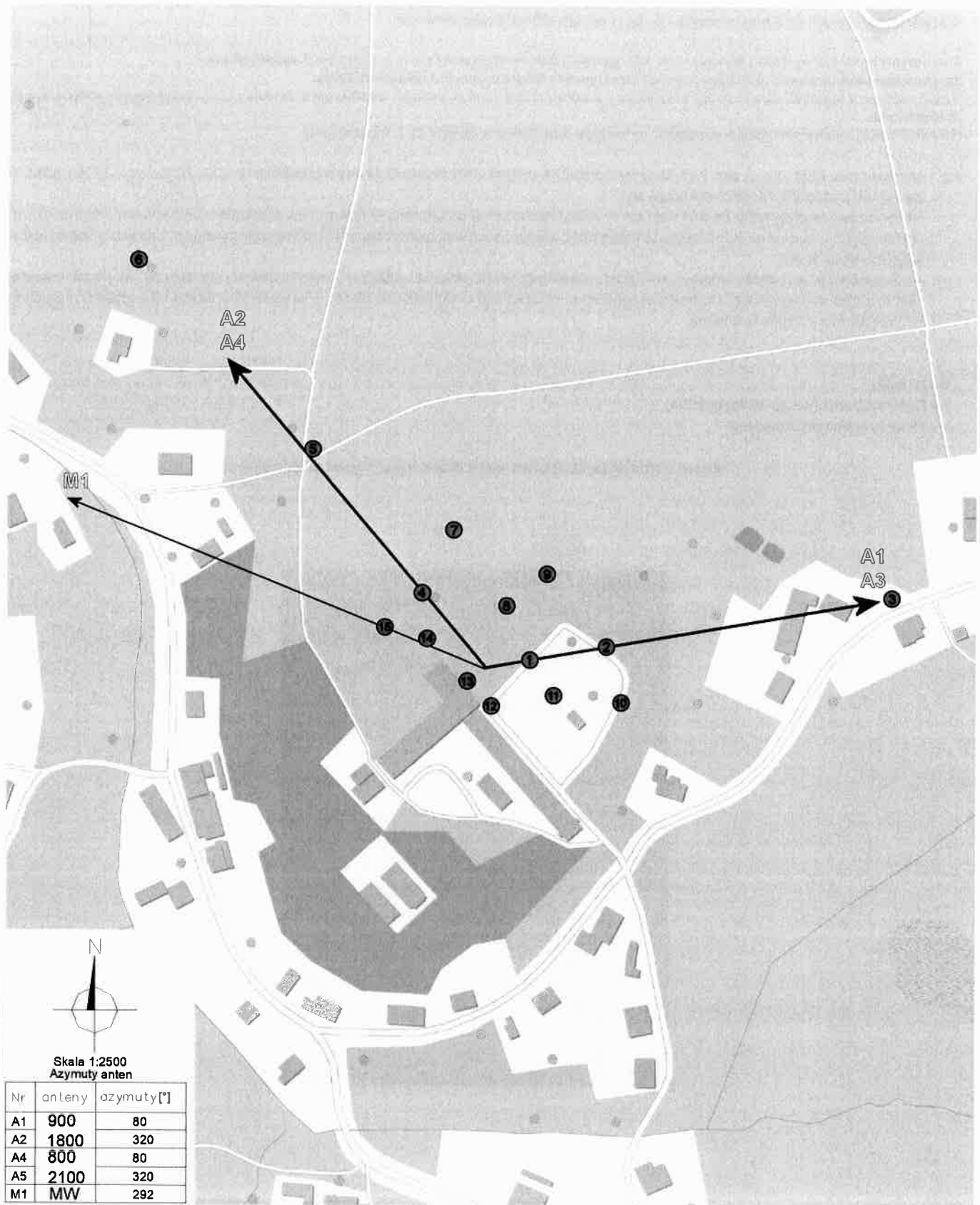
Zał. nr 2: Lokalizacja anten oraz ich azymuty, lokalizacja pionów (punktów) pomiarowych wokół instalacji radiokomunikacyjnej.
